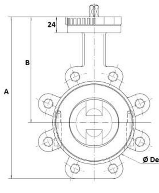
DN80-200
